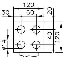
Připojovací kus FP M48x3
